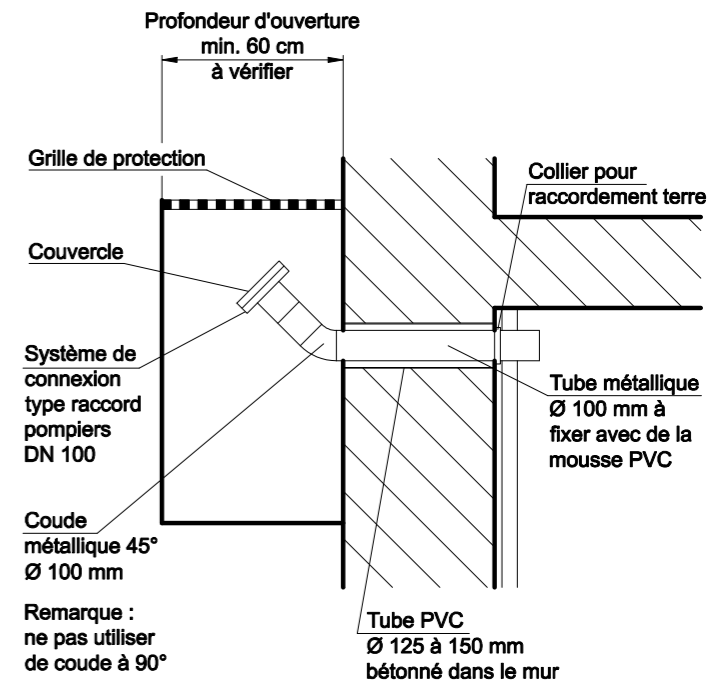
COUPE A Détail raccord de remplissage Echelle : 1/25
